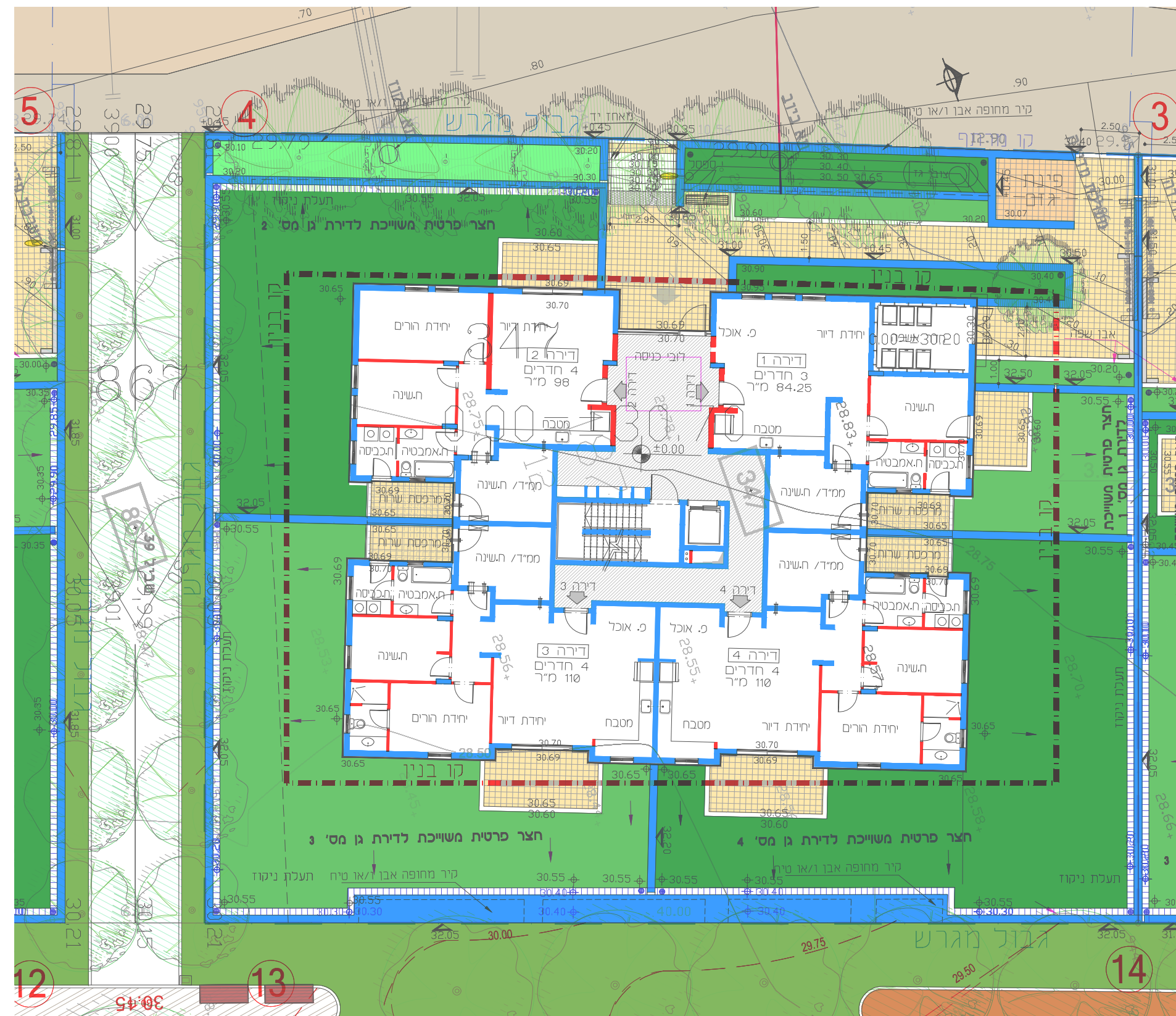
תכנית קומת קרקע קנ"מ 1:200
