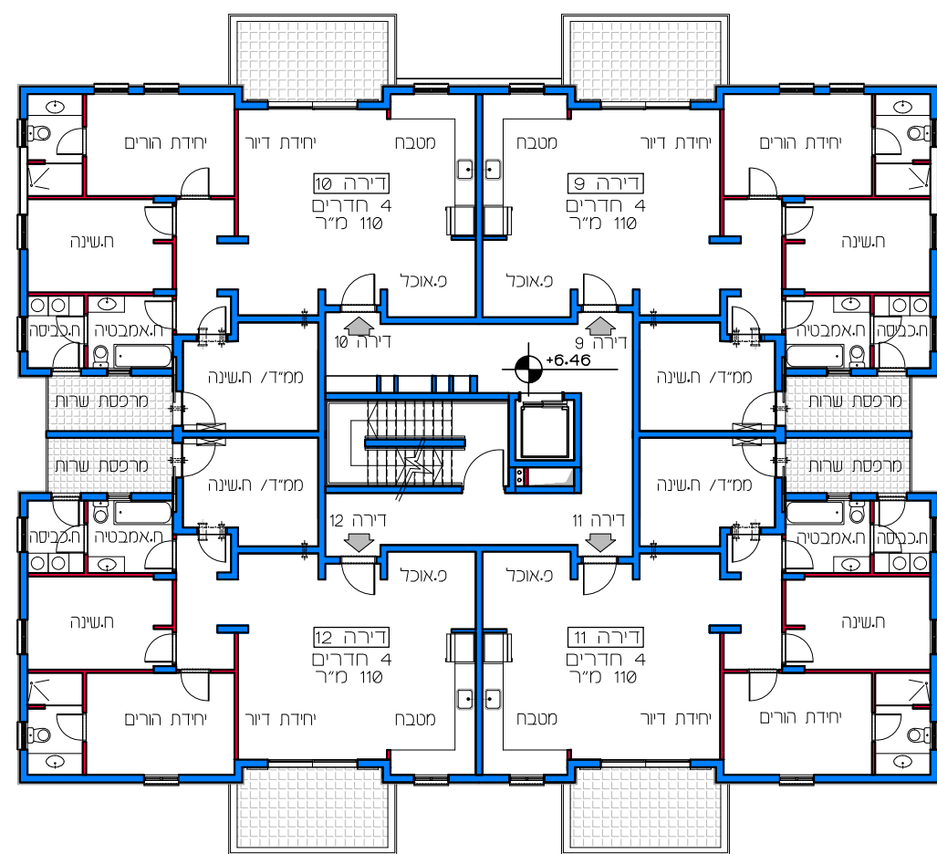
תכנית קומה 2 קנ"מ 1:200
